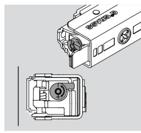
Store dører - anbefales maks demping
